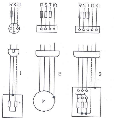
Şekil 12 - Elektrik tüketicilerinin sıfırlamada fiş ve priz üzerinden taşınabilir bağlantılarının yapılması
