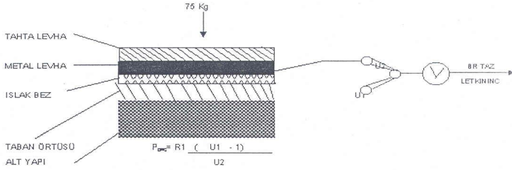
Şekil 20 – Zemin yalıtımlık direncinin ölçülmesi
