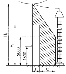
Şekil-7 Yere konulan normal çiti bulunan aygıtlarda koruma alanı
